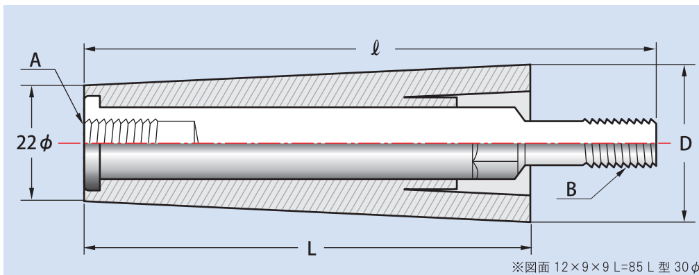
※図面 12×9×9 L=85 L型 30φ
